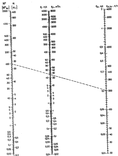
Черт. 4. Номограмма для определения секундных и часовых расходов воды в зависимости от NP (NP_{hr}) при различных значениях q_0 , л/с , q_{0,hr} , л/ч
