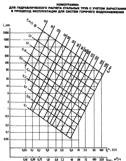
"Приложение 6. Номограмма для гидравлического расчета стальных труб с учетом зарастания в процессе эксплуатации для систем горячего водоснабжения"
