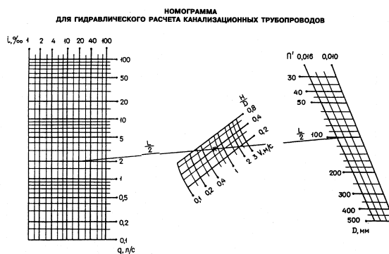
"Приложение 9. Номограмма для гидравлического расчета канализационных трубопроводов"
