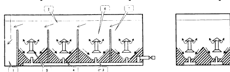
Рис. 4. Камера хлопьеобразования с малогабаритными аппаратами для рециркуляции осадка: 1 – отстойник; 2 – камера хлопьеобразования; 3 – канал исходной воды; 4 – трубопровод с осадком; 5 – емкостель; 6 – направляющий аппарат; 7 – перегородка
