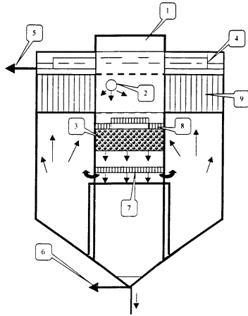
Рис. 1. Вертикальный тонкослойный отстойник с контактной камерой хлопьеобразования: 1 – крышка хлопьеобразования; 2 – подача исходной воды; 3 – контактная плавучая загрузка; 4 – сборный лоток; 5 – отвод осветленной воды; 6 – сбор осадка; 7, 8 – нижняя и верхняя поддерживающие решетки, соответственно; 9 – тонкослойные сотоблоки
