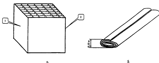
Рис. 6. Тонкослойный сотоблок из полиэтиленовой пленки: а – общий вид; б – в сложенном виде при транспортировке; 1 – тонкослойный блок из полиэтиленовой пленки; 2 – стержни для растяжения сотоблока
