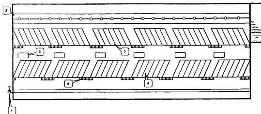
Рис. 2. Тонкослойный осветлитель, оборудованный тонкослойной камерой хлопьеобразования: 1 – подача исходной воды; 2 – сбор осветленной воды; 3 – пламеотводящие окна; 4 – тонкослойная камера хлопьеобразования; 5 – тонкослойные отстойные сотоблоки; 6 – поперечные опоры под блоки
