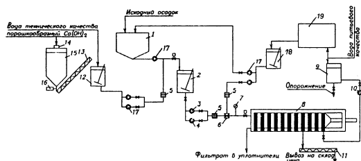
Рис. 10. Принципиальная технологическая схема обработки осадка на камерных фильтрах-прессах: 1 – уплотнитель исходного осадка; 2 – приемный резервуар осадка; 3 – насос быстрого заполнения; 4 – насос высокого давления; 5 – расходомер; 6 – узел сооплотителя; 7 – маломощный насос; 8 – камерный фильтр-пресс; 9 – резервуар воды для промывки фильтров-пресса; 10 – насос на промывку; 11 – плоский транспортер; 12 – резервуар базовых реагентов; 13 – плоский транспортер; 14 – фильтр; 15 – силосная башня; 16 – вибратор; 17 – плоский насос-дозатор; 18 – расходный бак флокулянта; 19 – узел приготовления раствора флокулянта
