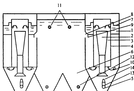
Рис. 8. Осветлитель-рециркулятор:
