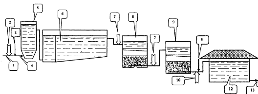
Рис. 9. Применение озона и активных углей на станциях с двухступенной схемой очистки воды: 1 - подача речной воды; 2 - первичное озонирование; 3 - первичное хлорирование (при необходимости); 4 - зона коагулянта; 5 - осветлитель; 6 - отстойник (для окисляемых органических веществ); 7 - вторичное озонирование; 8 - песчаный фильтр; 9 - угольный фильтр; 10 - третичное озонирование; 11 - вторичное хлорирование; 12 - резервуар чистой воды; 13 - подача питьевой воды потребителю
