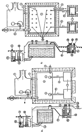
Рис. 8. Устройство герметизированных резервуаров питьевой воды с фильтрами-поглопителями и площадками для сбора воды a — эксплуатируемый резервуар; b — вновь проектируемый резервуар; 1 — площадка запорно-защитная и инвентарная; 2 — ступенчатый трубопровод; 3 — герметичный док-лак; 4 — подающий трубопровод; 5 — резервуар питьевой воды; 6 — воздуховод; 7 — камера фильтров-поглопителей; 8 — отводящий трубопровод; 9 — патрубок с фланцевой заглушкой; 10 — колодец на отводящем трубопроводе с арматурой; 11 — мокрый колодец с герметичным доком; 12 — аварийный стоик; 13 — стоик для выпуска воздуха; 14 — стоик для выпуска воздуха; 15 — фильтр-поглодитель; 16 — камера фильтра-поглопителя; 17 — пожарный гидрант со стенодером; 18 — вентиляционные колонки
