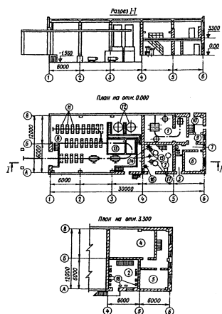
Рис. 11. Устройство хлораторной с повышенной надежностью
