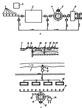
Рис. 2. Принципиальные технологические схемы сооружений
