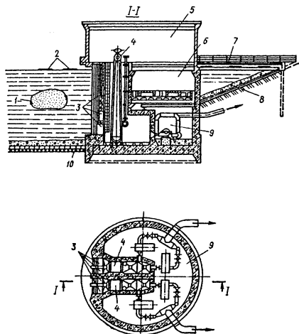
Рис. 5. Водозаборы из поверхностных водоисточников 1 – мигрирующий слой планктона; 2 – плавающие пленки; 3 – водоприемные окна с плоскими сетками; 4 – вращающиеся сетки; 5 – наземный павильон; 6 – помещение для электрооборудования; 7 – мост; 8 – береговые отложения; 9 – машинный зал; 10 – донные осадки
