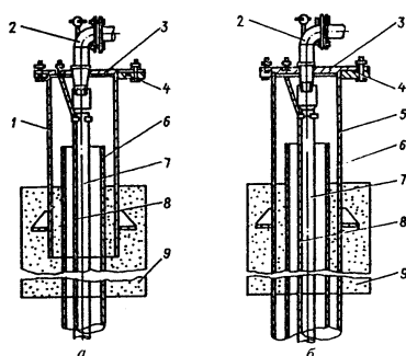
Рис. 3. Устройство герметизированных оголовков артскважин
