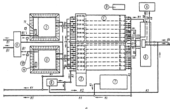
Рис. 7. Схема устройств для приготовления и дозирования реагентов на водоочистных станциях при двухступенчатой схеме очистки
