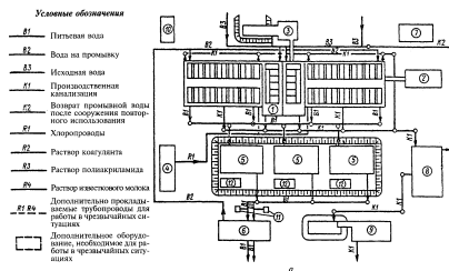
Рис. 6. Схема устройств для приготовления и дозирования реагентов на водоочистных станциях при одноступенчатой схеме очистки
