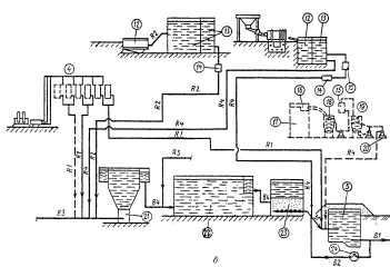
Рис. 7. Схема устройств для приготовления и дозирования реагентов на водоочистных станциях при двухступенчатой схеме очистки
