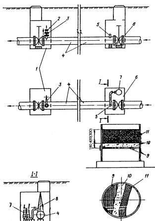
Рис. 9. Устройства для отбора питьевой воды из водоводов и магистральных трубопроводов систем подачи и распределения воды 1 — колодец для отбора воды в пониженных точках сети, 2 — патрубков, 3 — задвижка, 4 — магистральный трубопровод, 5 — выпуск воздуха через фильтр-поглонитель, 6 — колодец с фильтром-поглодителем в повышенных точках сети, 7 — фильтр-поглонитель из местных материалов, 8 — воздуховод, 9 — металлическая решетка, 10 — трамвайная загрузка, 11 — фильтрующий слой
